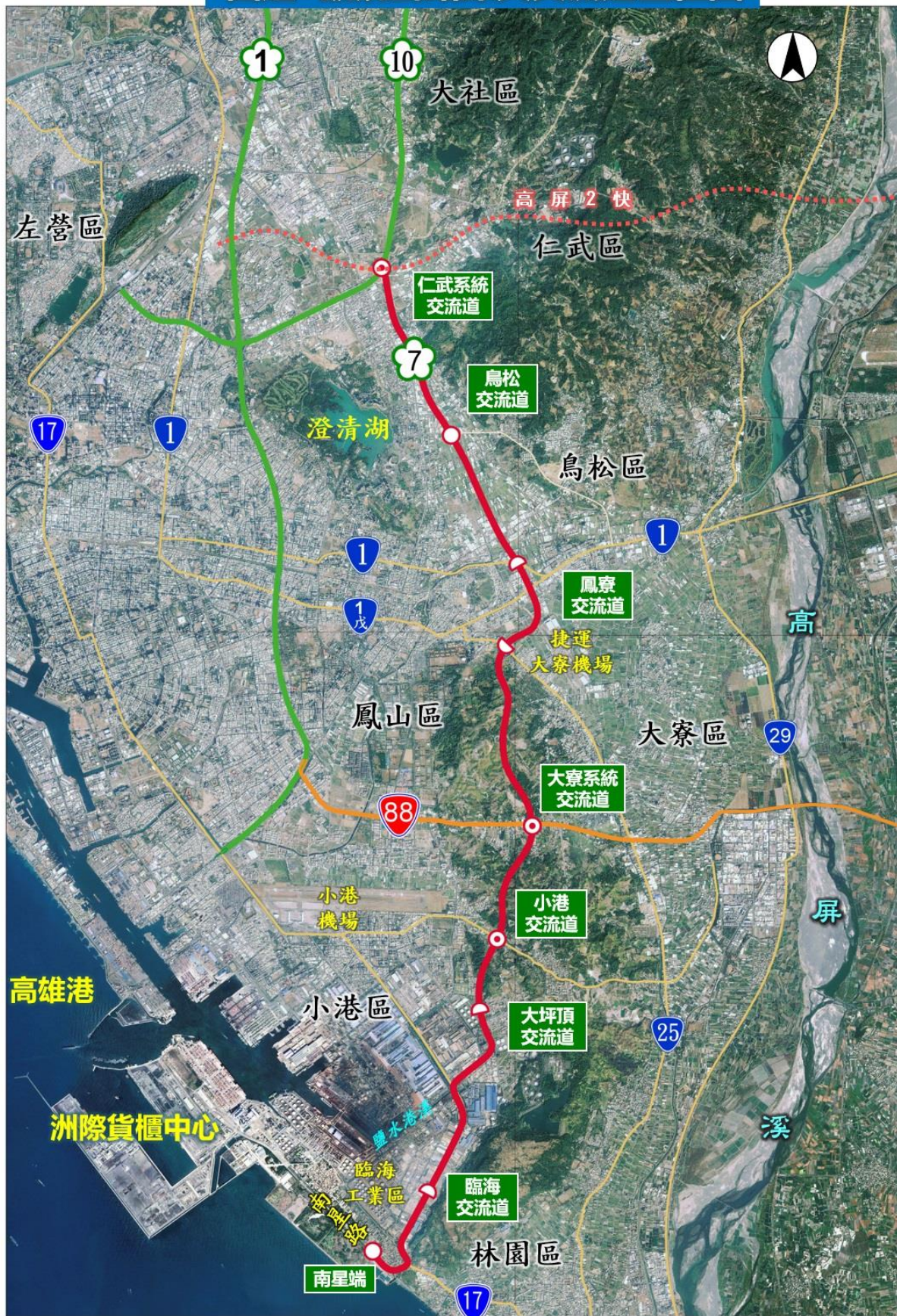
附圖 國道7號高雄路段計畫示意圖
